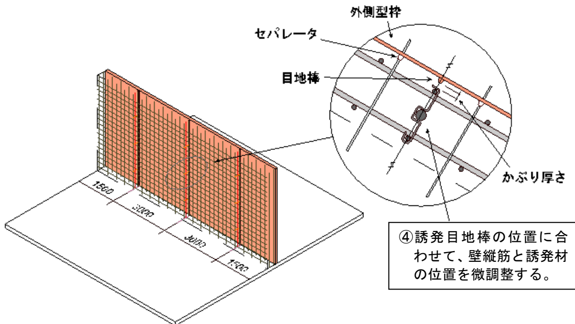
図-4 施工手順図3
