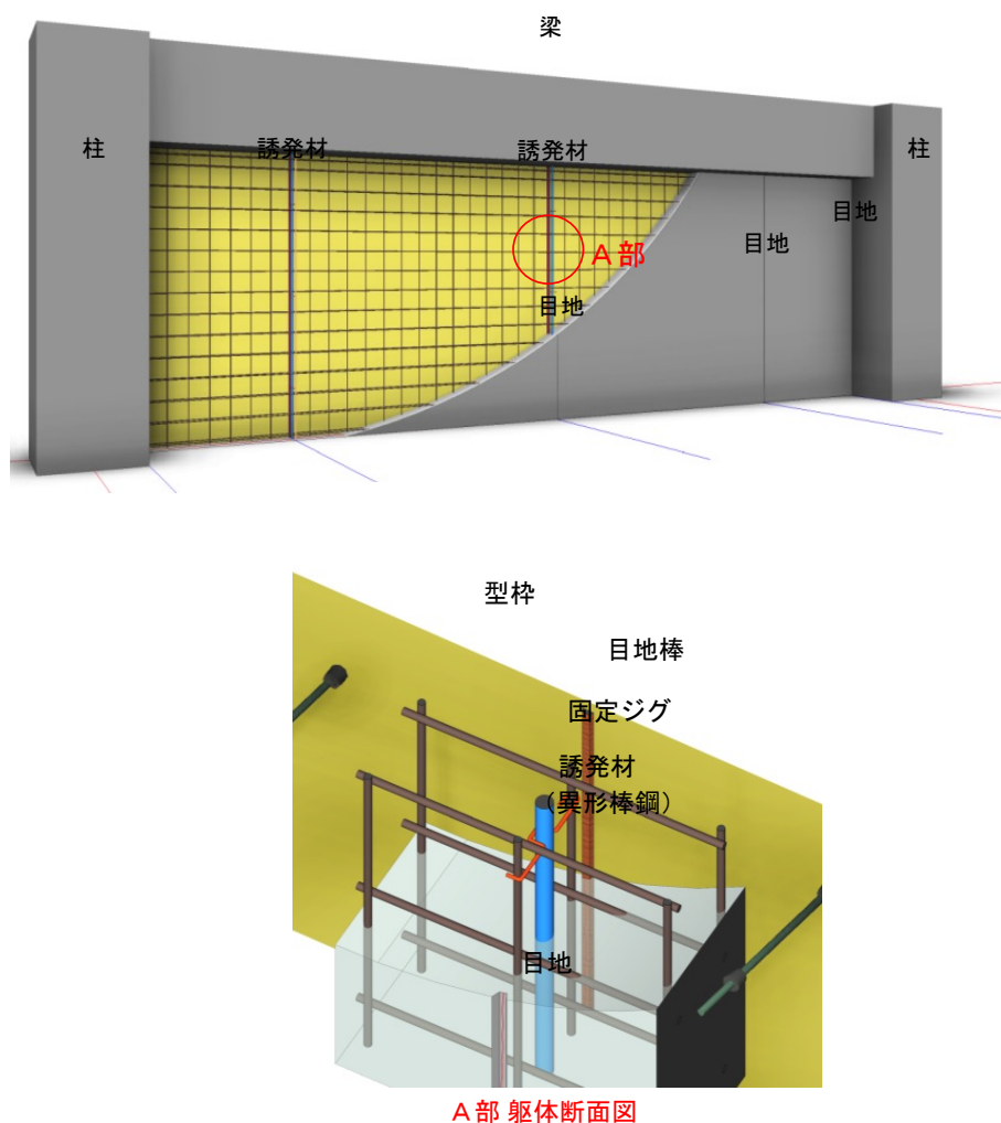
図-1 CCB工法概要図
